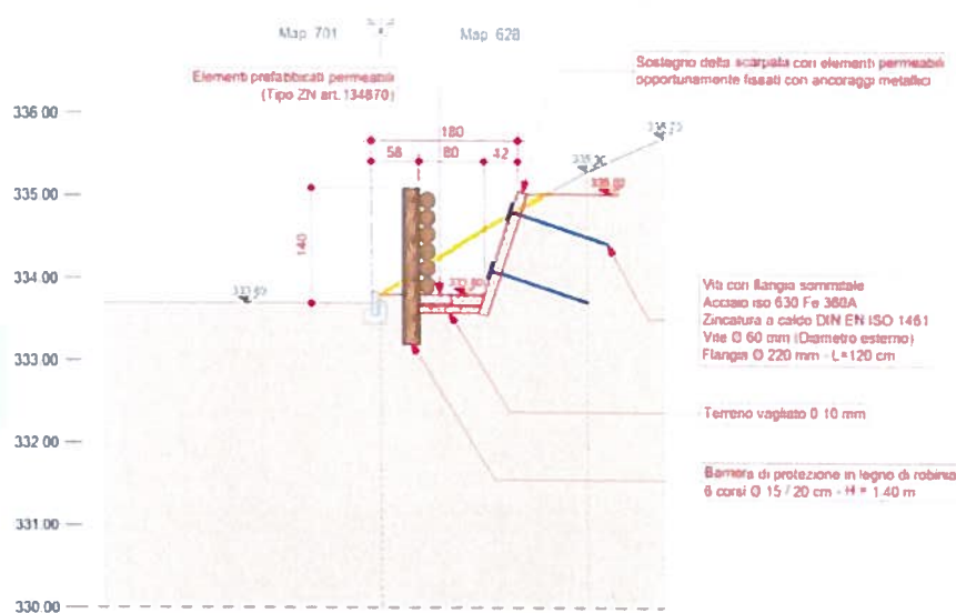
Elemento puntuale di stabilizzazione Sezione tipo 1:50
